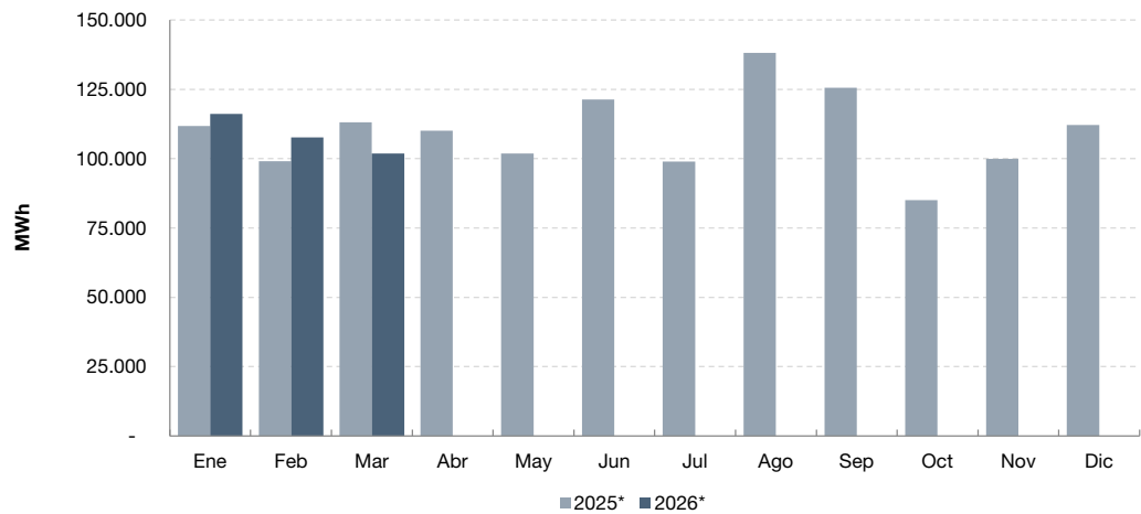
Gráfico 2.4 Energía cogenerada total en MWh. Industria manufacturera. Enero 2025-marzo 2026
