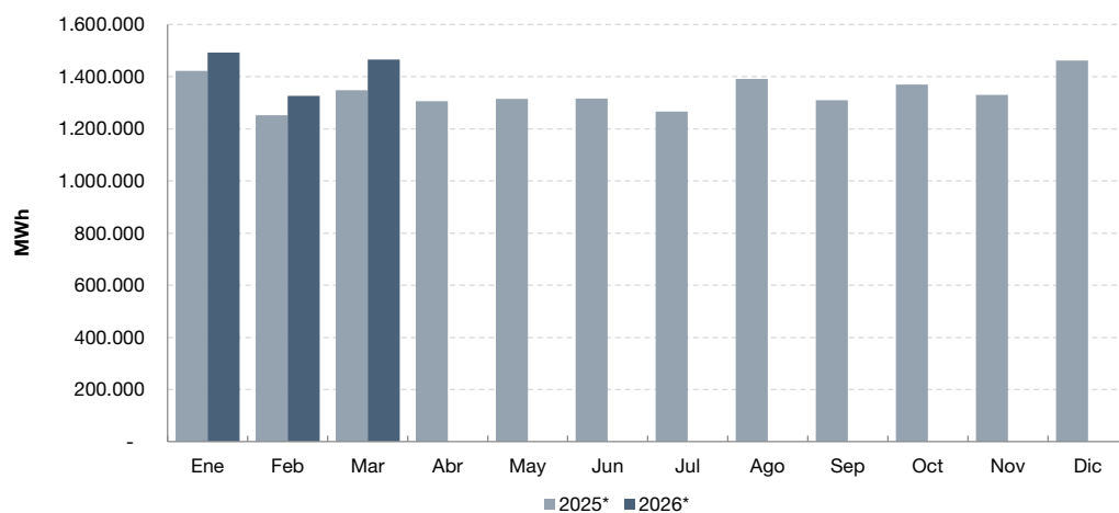
Gráfico 2.2 Energía autogenerada despachada al MEM en MWh. Minería e industria manufacturera. Enero 2025-marzo 2026
